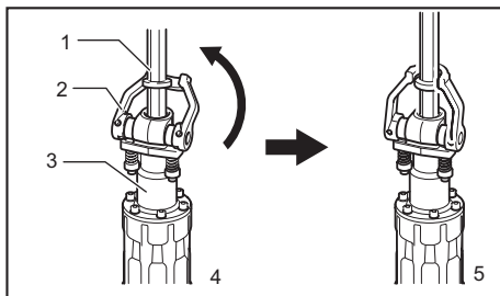
► 1. Embout 2. Dispositif de retenue 3. Porte-outil 4. Lorsque le foret est inséré 5. Lorsque le foret est retenu
