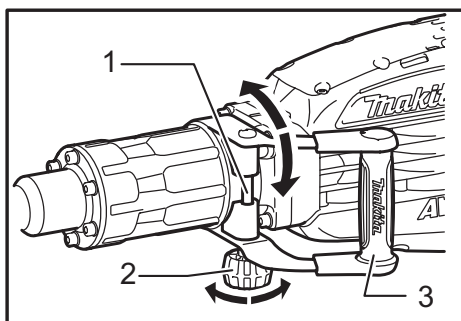
► 1. Boulon 2. Écrou 3. Poignée étrier latérale
